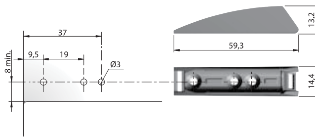
Schemat wierceń i wymiary adaptera dla wersji 14 mm
