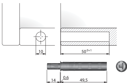
Schemat wierceń dla wersji wpuszczanej
